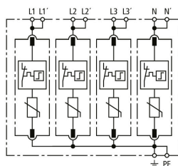
Prinzipialschaltbild DG MP TNS 275
