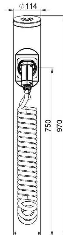
electrify eSat r20 Ladesäule, links: 3D Modell; rechts: Abmessungen (Maßeinheit mm)
